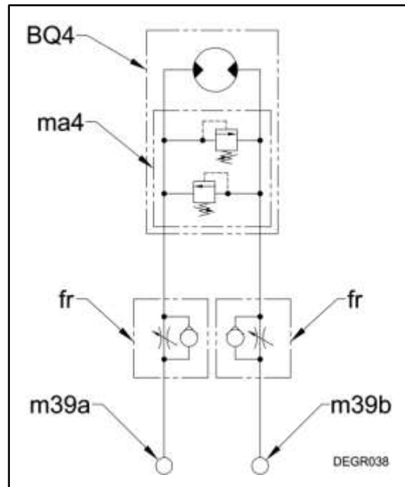
CIRCUITO HIDRÁULICO CON MOTOR SIMPLE
